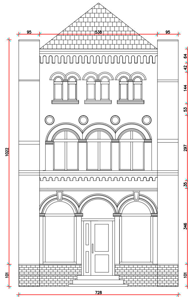
Elewacja frontowa
