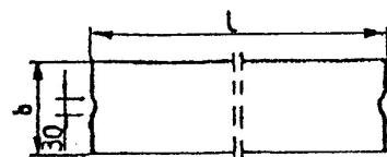
c) wpusty na powierzchniach stykowych krawężników
