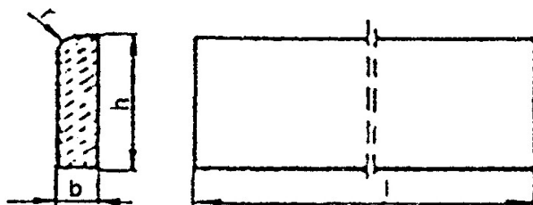
Rysunek 1. Kształt betonowego obrzeża chodnikowego
