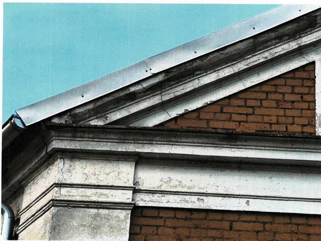
GZYMS WIENĆZĄCY Z GZYMSEM PRZY POŁACI DACHOWEJ
